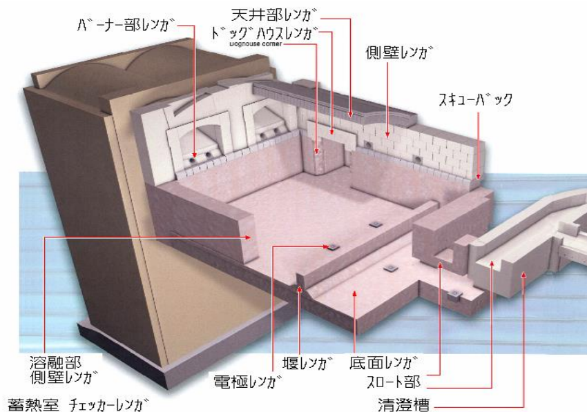
ガラス溶解炉レンガ構成例
